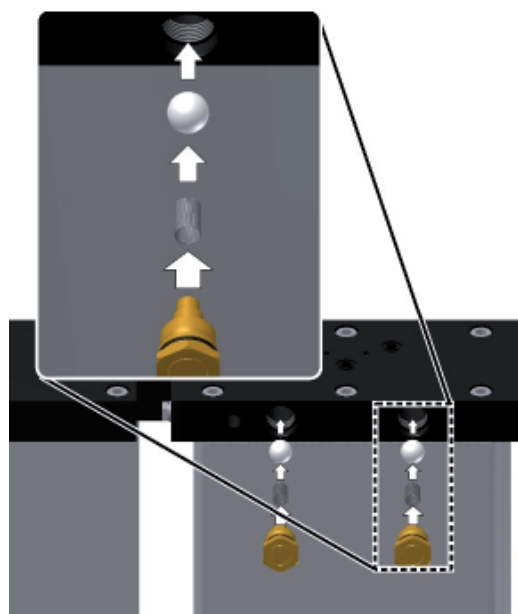
Zpětné ventily
